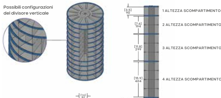
Dimensioni dei compartimenti in base alla configurazione
